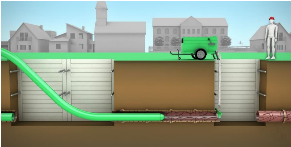
Abbildung 3: Rohrstrangverfahren
